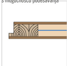
KRILU 46 mm ojačano čeličnim limom
